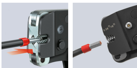
Čelní zavádění dutinek např. ve skříňových rozvaděčích
