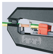
precizní odizolování od 0,2 - 6,0 mm 2
