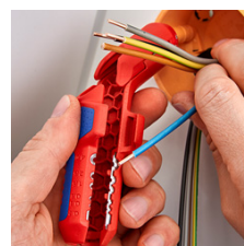
Odizolování jednotlivých vodičů
