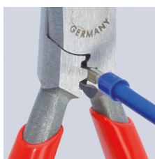
Krimpování 0,5 až 2,5 mm 2
